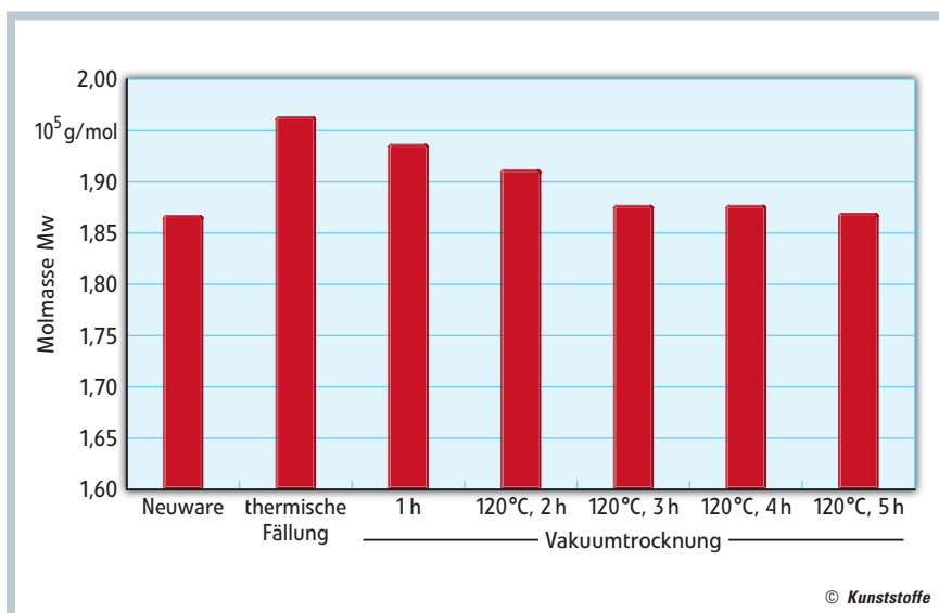
Bild 5. Molmassenerhalt und Aufbau von PLA bei verschiedenen Löse-/Fäll- und Trocknungsbedingungen mittels CreaSolv-Prozess (Bild: Fraunhofer IVV)
