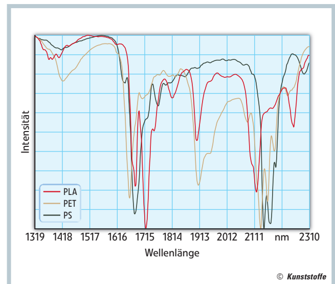
Bild 2. NIR-Spektren von PLA, PET, PS
